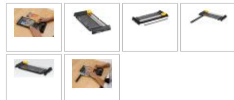
Neutrino
